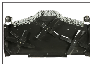
Mulchmäherwerk 110 cm
